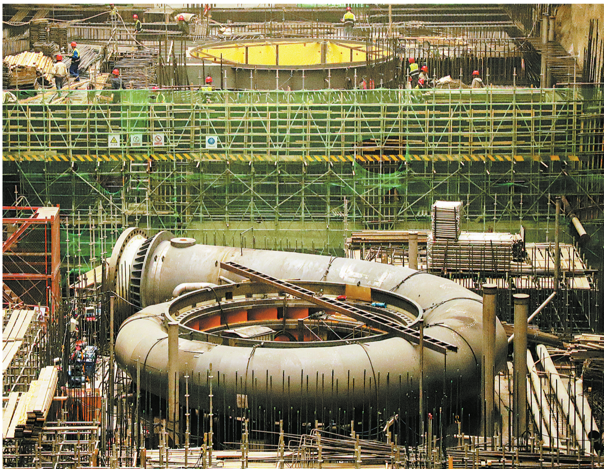
镇安抽水蓄能电站位于镇安县月河镇，是我国西北地区开工建设的首个抽水蓄能电站工程。该电站设计年发电量23.41亿千瓦时，以330千伏电压接入陕西电网。项目建成后，将有力地增强陕西电网灵活调节和抵御事故风险能力，可带动GDP增长约45亿元。（本报记者 米子扬 摄）
