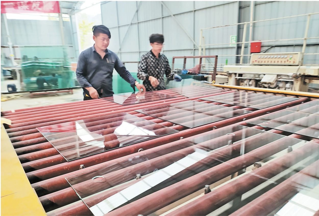
6月23日,工人在商洛市艺海远玻璃公司车间裁制玻璃制品。该公司位于商州区杨镇镇松云创新创业示范基地,是一家社区工厂,现有员工50人。公司主要生产加工幕墙装饰玻璃、家居日用玻璃等,年产值1500万元,安置当地30多名劳动力进厂就业,人均月收入3500元以上。(本报记者 贾书章 摄)
